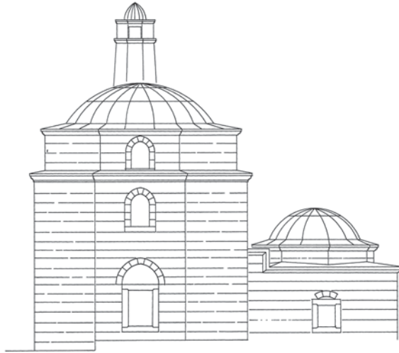
BATI CEPHE 1/50
