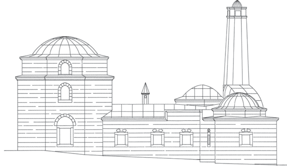
GÜNEY CEPHE 1/50
