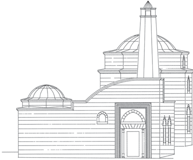
DOĞU CEPHE 1/50
