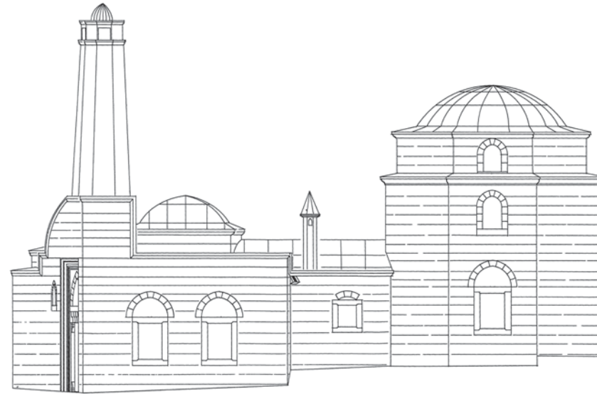
KUZEY CEPHE 1/50
